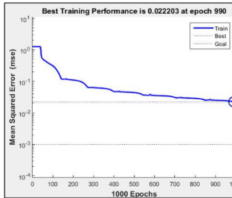
Gambar 10. Nilai MSE
