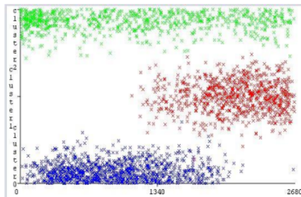
Gambar 6. Visualisasi Hasil
