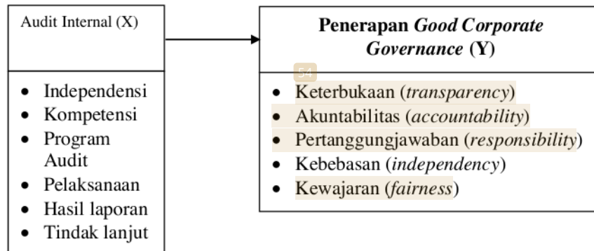
Gambar 1. Kerangka Penelitian
