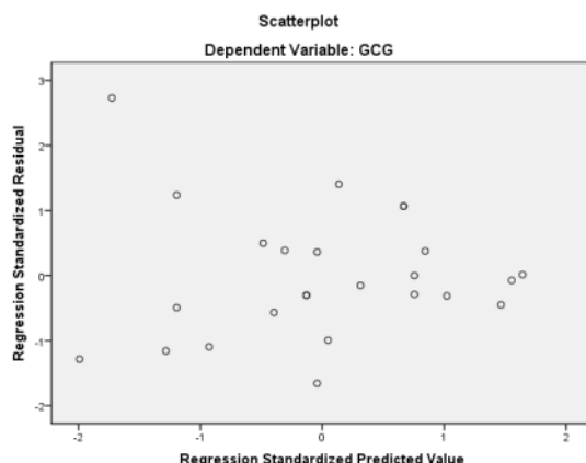
Gambar 3. Grafik Scatterplot
