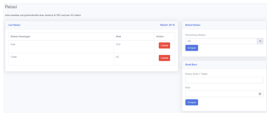
Gambar 8. Formulir relasi
