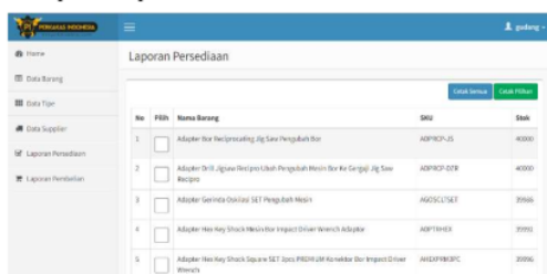
Gambar 12. Tampilan Laporan Persediaan
