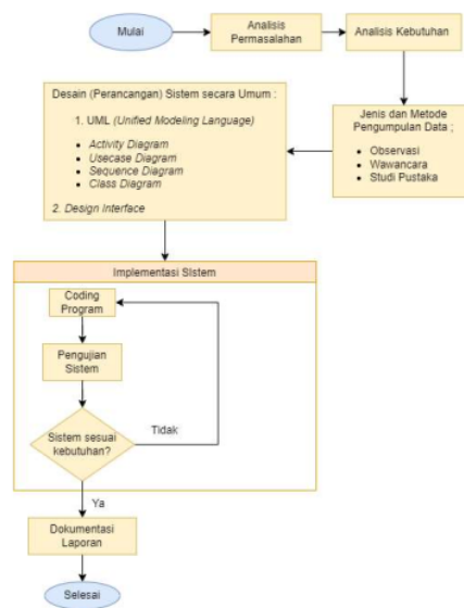
Gambar 1. Metodologi Penelitian
