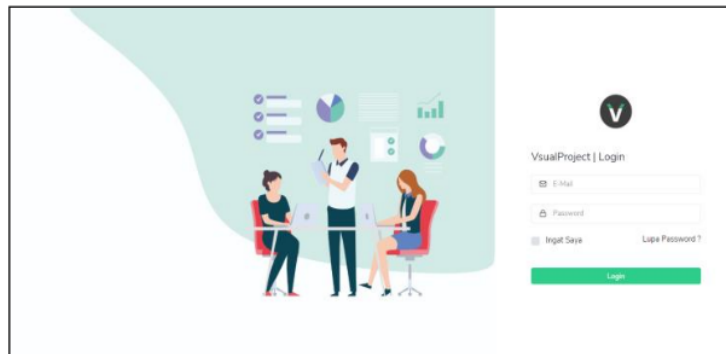
Gambar 4. Halaman Login
