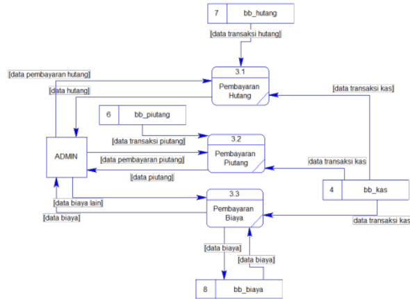
Gambar 5. DFD level 1 Pembayaran
