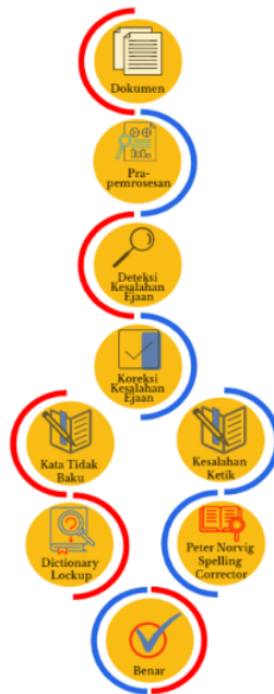
Gbr 1. Usulan perancangan desain sistem penelitian KEBI 1.0 Checker
