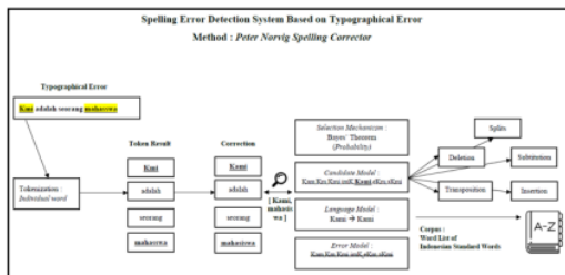
Gbr 3. Desain sistem proses deteksi kesalahan ejaan kata typo menggunakan metode Peter Norvig Spelling Corrector
