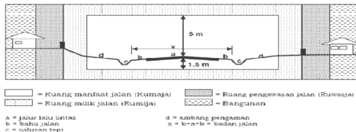
Gambar 1.1 Bagian – Bagian Jalan
