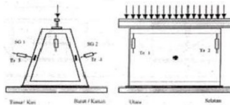
Gambar 1.2 Pondasi (Sumber: Nawir R.,2010)
