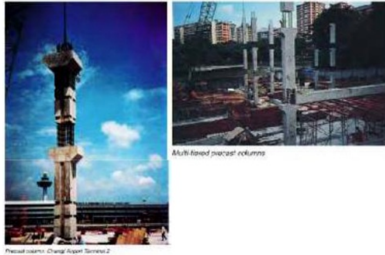
Gambar 1.6 Kolom Precast
