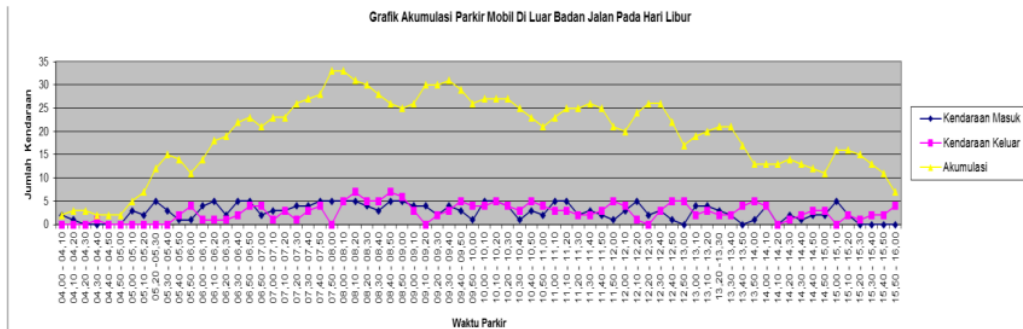
Gambar 2. Grafik Data Arus Kendaraan Mobil Di Luar Badan Jalan Hari Libur
