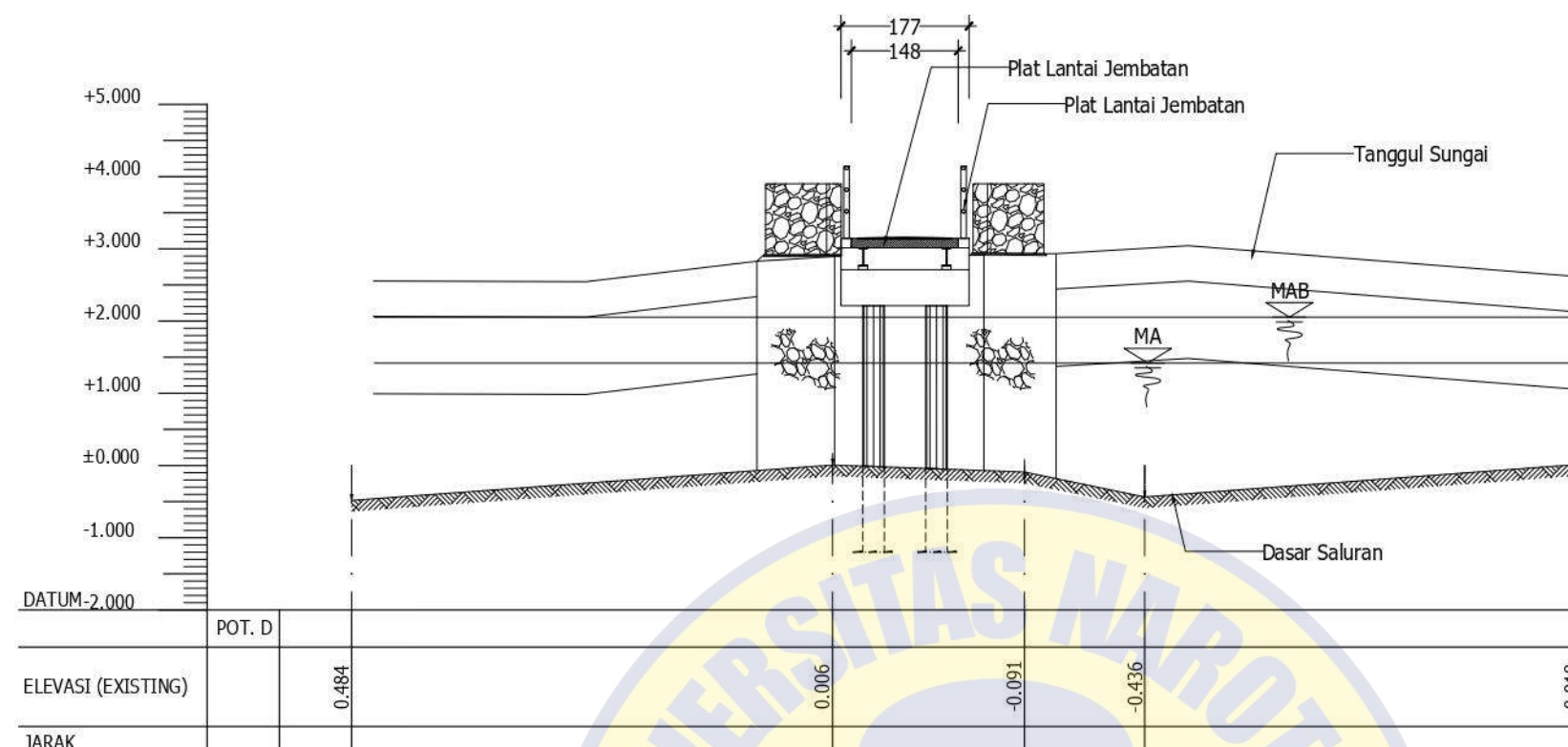
POTONGAN D-D (EXISTING) Skala 1 : 100
