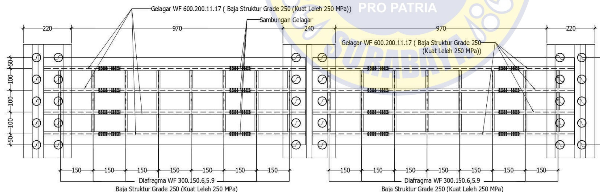
DENAH GELAGAR DAN DIAFRAGMA
