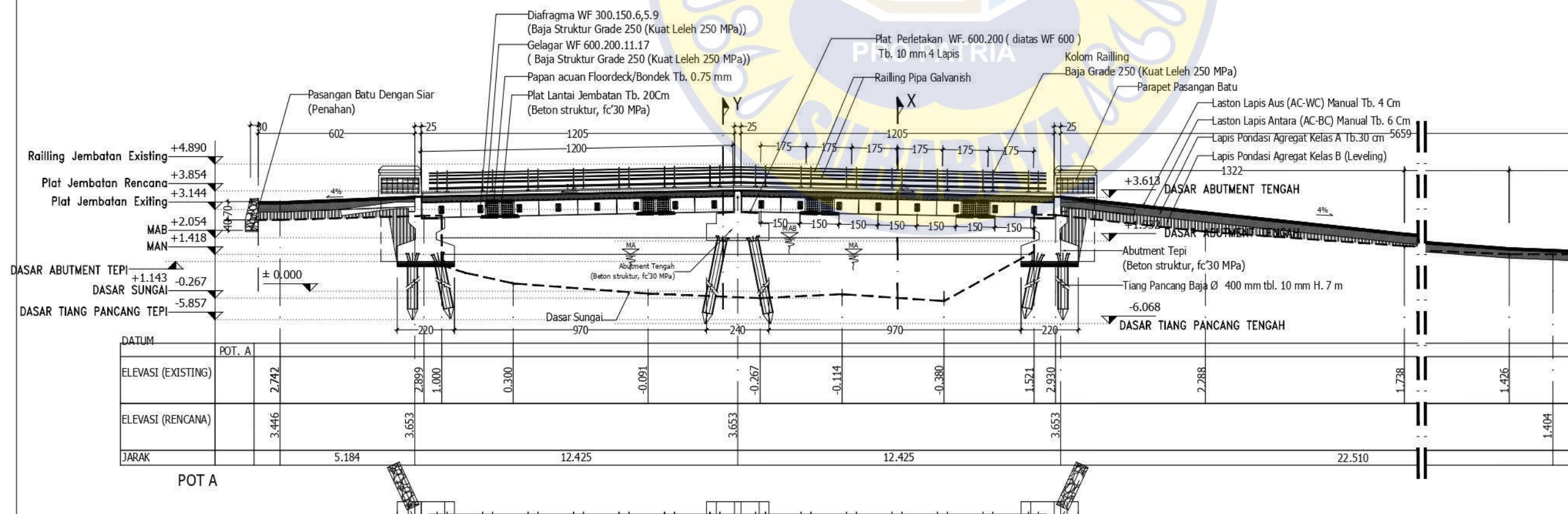
POTONGAN A-A (RENCANA) Skala 1 : 175
