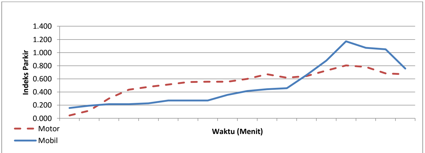
Gambar 4.7d Grafik Indeks Parkir Motor&Mobil Hari Selasa 5 Juli 2018
