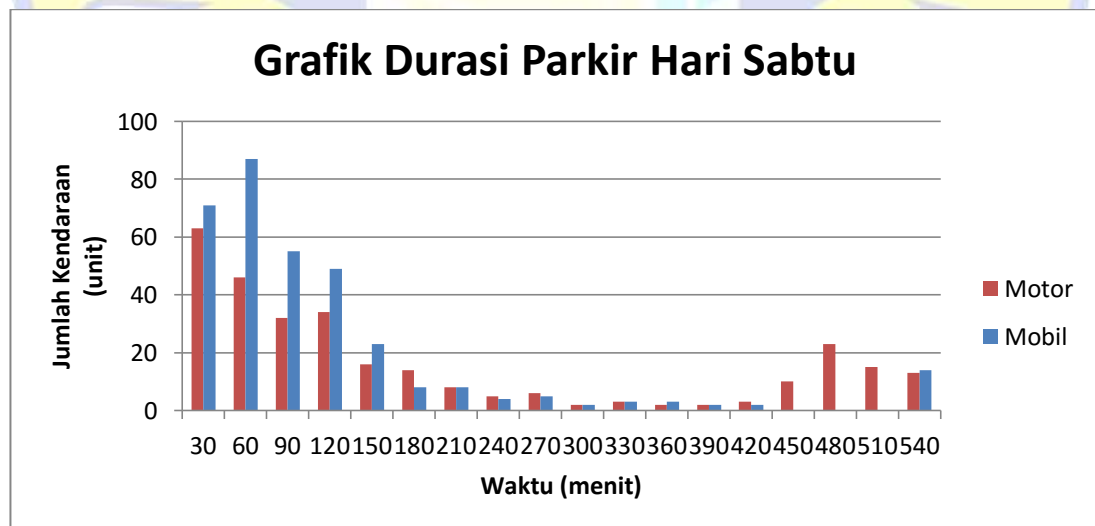
Gambar 4.1f Grafik Klasifikasi Durasi Parkir Hari Sabtu 2 Juli 2018
