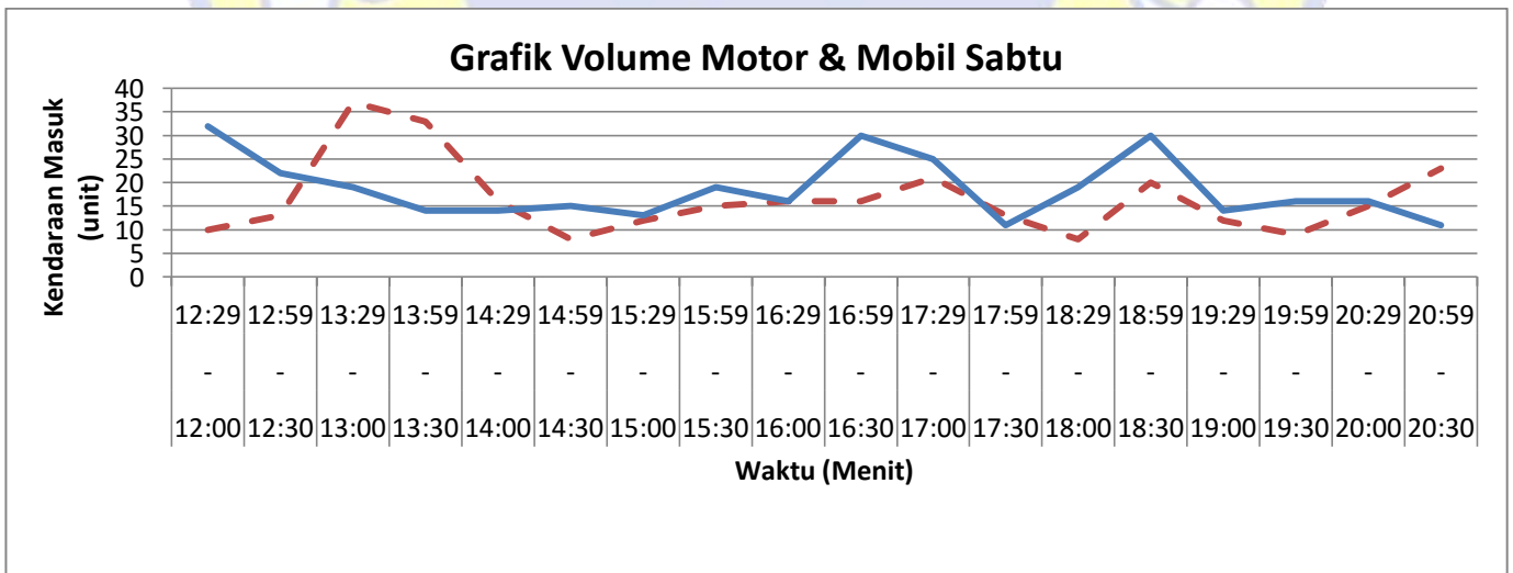
Gambar 4.3a Grafik Volume Sepeda Motor Dan Mobil Hari Sabtu 2 Juli 2018
