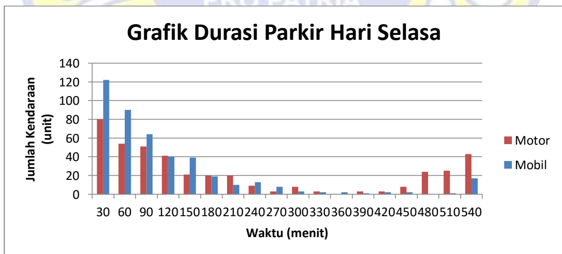
Gambar 4.1i Grafik Klasifikasi Durasi Parkir Hari Selasa 5 Juli 2018
