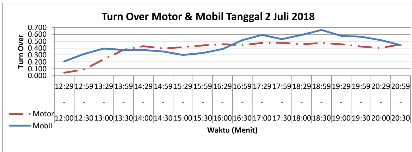
Gambar 4.5a Grafik Turn Over Sepeda Motor Dan Mobil Hari Sabtu 2 Juli 2018
