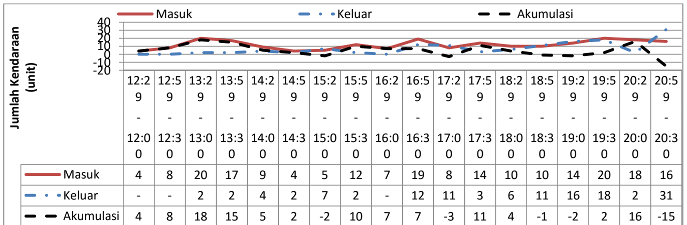
Gambar 4.2 Grafik Akumulasi Sepeda Motor Hari Jumat 1 Juli 2018
