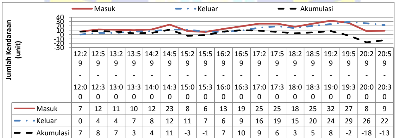
Gambar 4.2e Grafik Akumulasi Parkir Mobil Hari Minggu 3 Juli 2018
