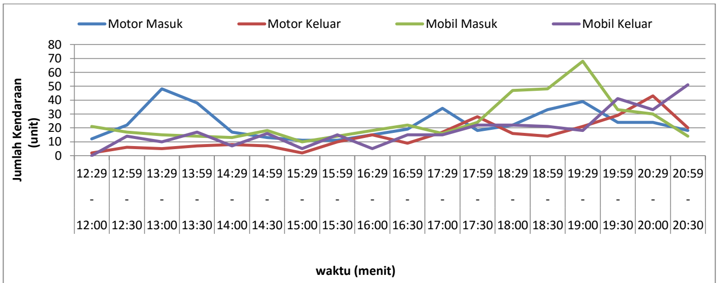
Gambar 4.1c Grafik Data Arus Kendaraan Hari Senin 4 Juli 2018
