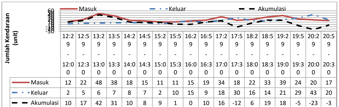
Gambar 4.2h Grafik Akumulasi Parkir Sepeda Motor Hari Selasa 5 Juli 2018
