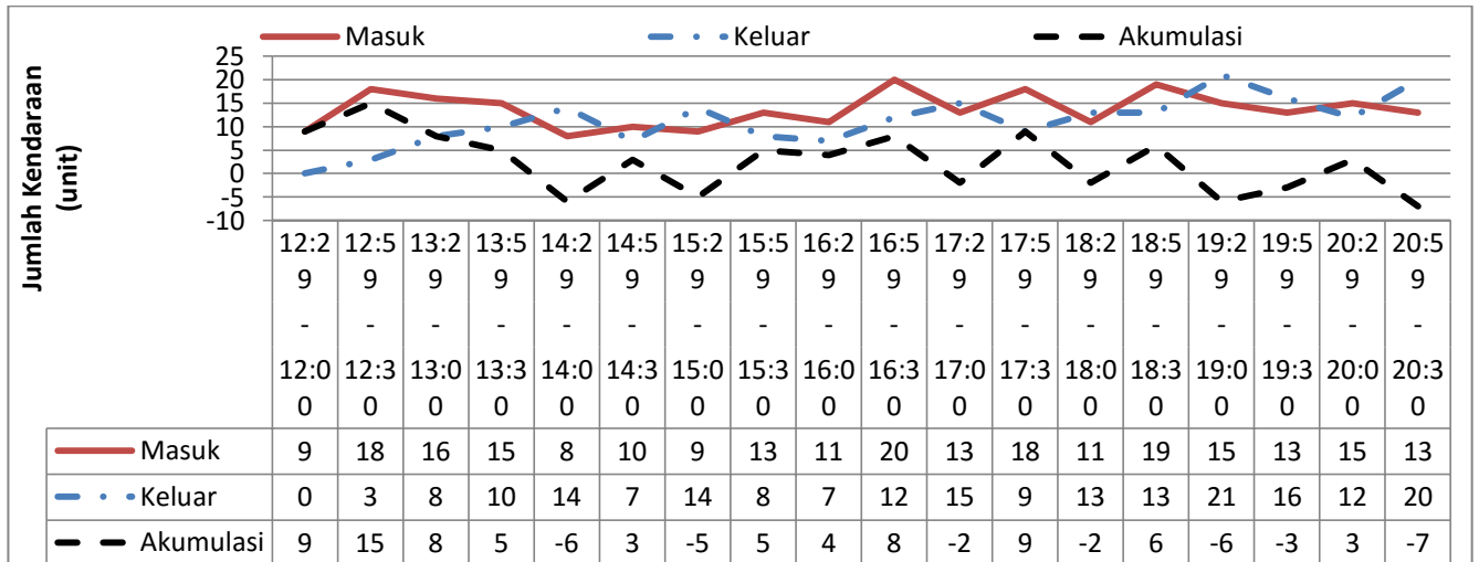
Gambar 4.2a Grafik Akumulasi Parkir Mobil Hari Jumat 1 Juli 2018
