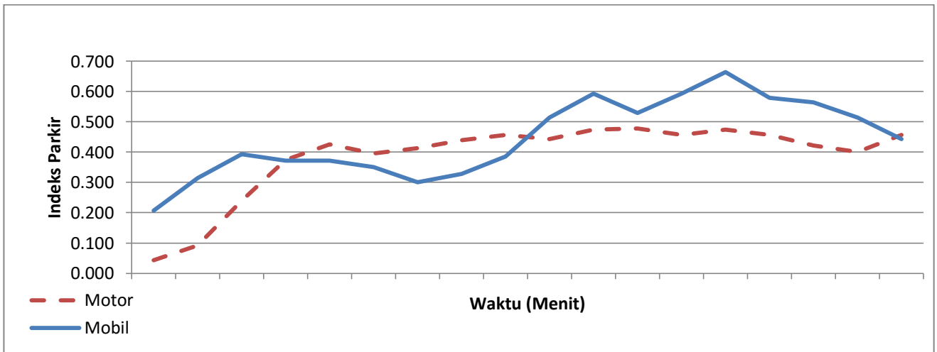
Gambar 4.7a Grafik Indeks Parkir Motor&Mobil Hari Sabtu 2 Juli 2018
