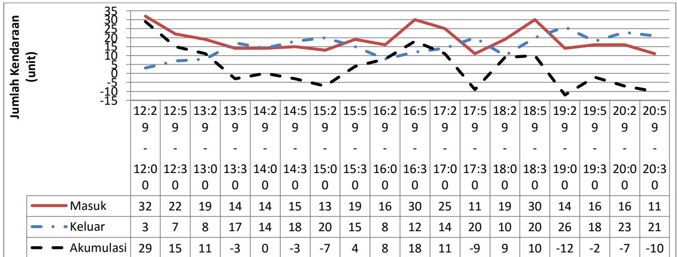
Gambar 4.2c Grafik Akumulasi Parkir Mobil Hari Sabtu 2 Juli 2018
