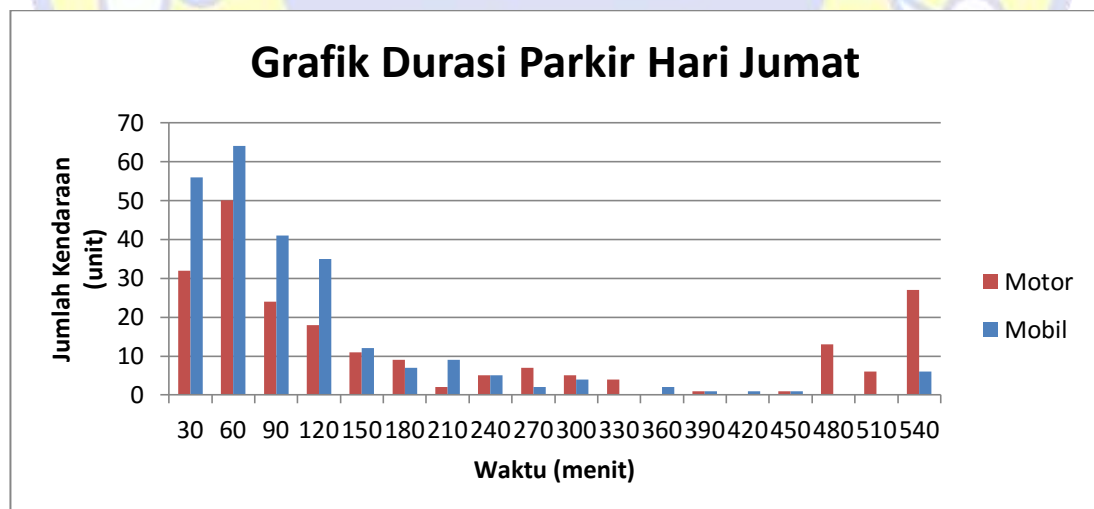
Gambar 4.1e Grafik Klasifikasi Durasi Parkir Hari Jumat 1 Juli 2018
