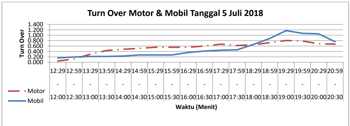
Gambar 4.5d Grafik Turn Over Sepeda Motor Dan Mobil Hari Selasa 5 Januari 2018
