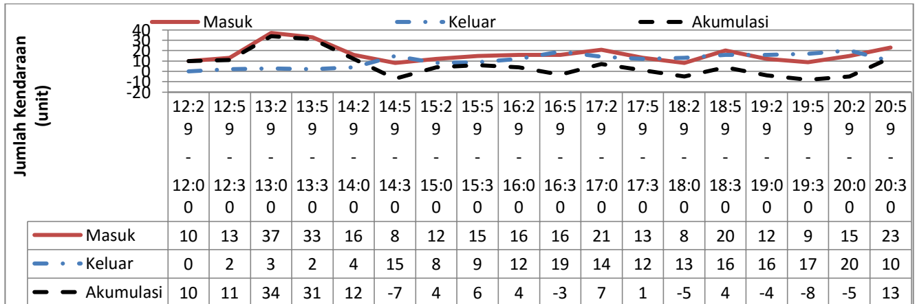
Gambar 4.2b Grafik Akumulasi Parkir Sepeda Motor Hari Sabtu 2 Juli 2018
