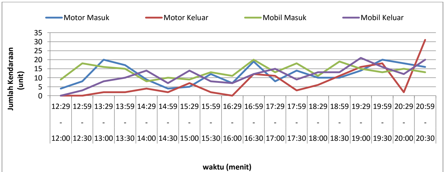
Gambar 4.1 Grafik Data Arus Kendaraan Hari Jumat 1 Juli 2018
