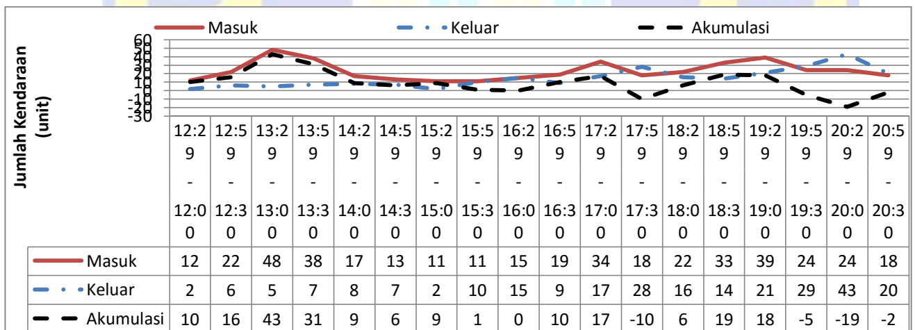
Gambar 4.2f Grafik Akumulasi Parkir Sepeda Motor Hari Senin 4 Juli 2018
