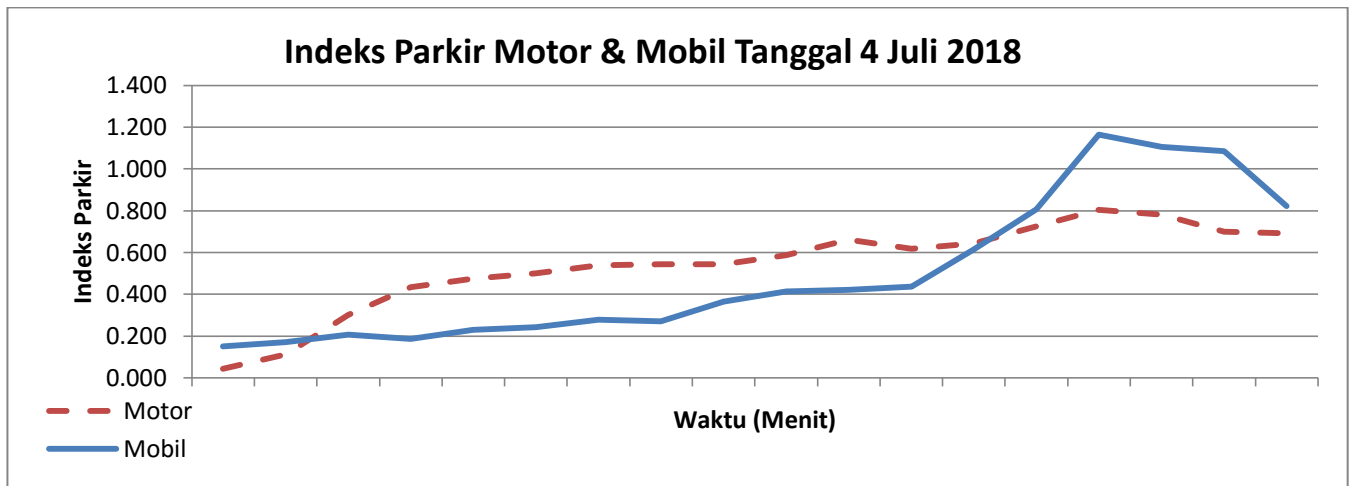
Gambar 4.7c Grafik Indeks Parkir Motor&Mobil Hari Senin 4 Juli 2018
