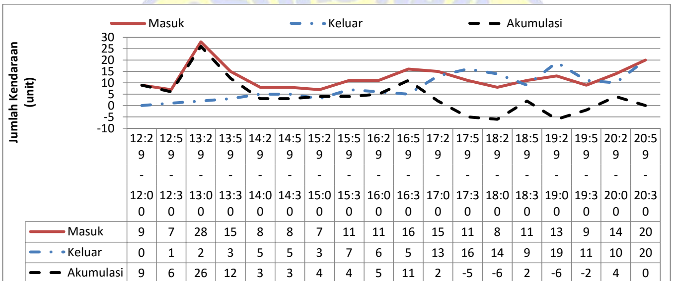
Gambar 4.2d Grafik Akumulasi Parkir Sepeda Motor Hari Minggu 3 Juli 2018
