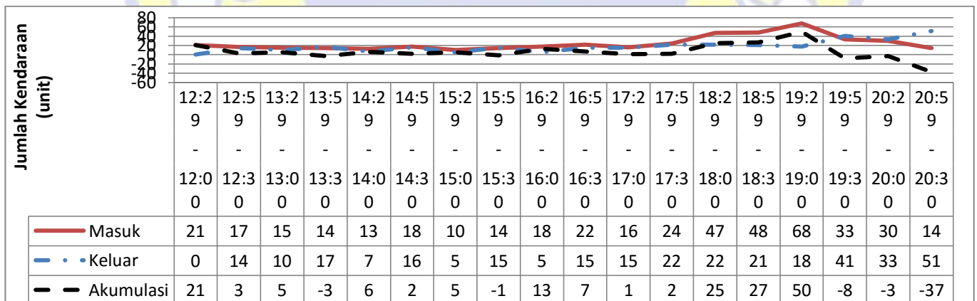
Gambar 4.2g Grafik Akumulasi Parkir Mobil Hari Senin 4 Juli 2018
