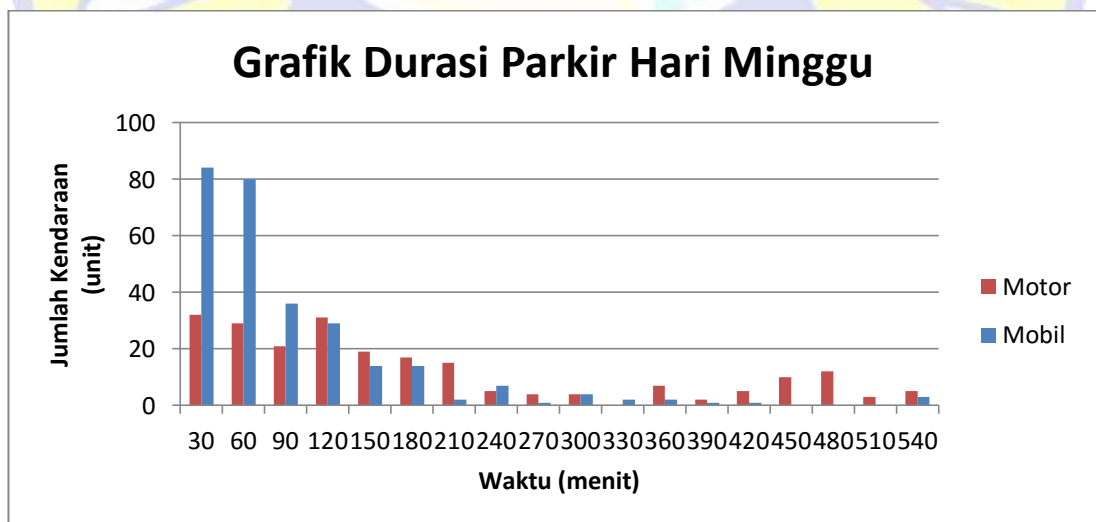
Gambar 4.1g Grafik Klasifikasi Durasi Parkir Hari Minggu 3 Juli 2018
