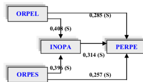
Gambar: 1 Diagram Path Hasil Pengujian Koefisien Jalur
