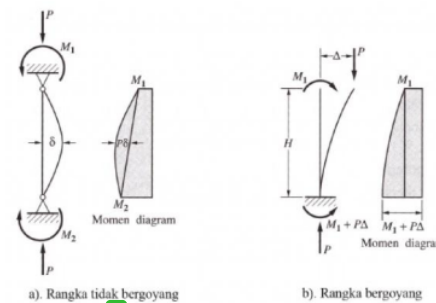
Gambar 4. Momen yang dipengaruhi Efek P-delta
